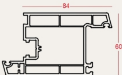
Casement Door Sash Inward SBM-CS-005
