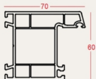
Casement Door Frame 60mm SBM-CS-006
